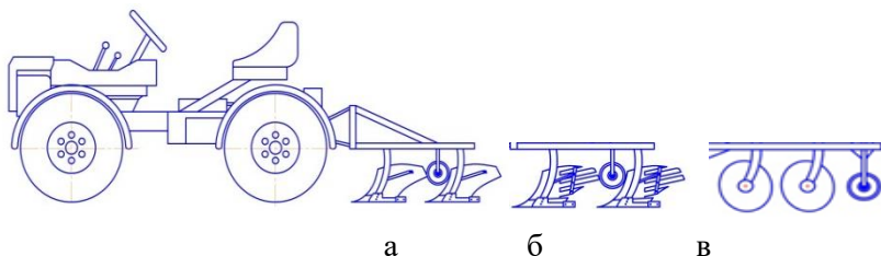
Рисунок 3 – Мини-трактор + плуг с цилиндрическим отвалом (а), пластинчатым отвалом (б), дисковый плуг (в)
