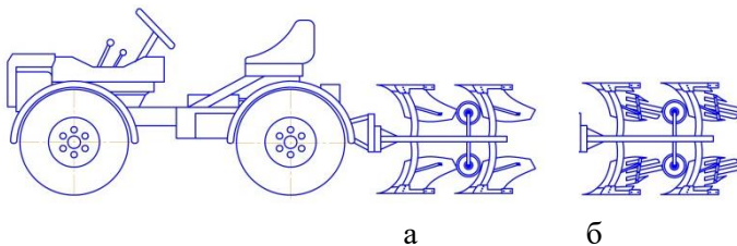
Рисунок 4 – Мини-трактор + оборотный плуг с цилиндрическим (а) и пластинчатым отвалом (б)
