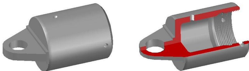
Рисунок 2. Пример построения модели корпуса пневмоцилиндра
