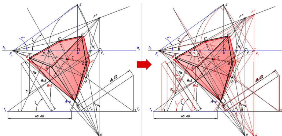
Рисунок 4 – Проверка: неверное выполнение задания
