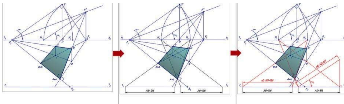
Рисунок 5 – Проверка решения метрической задачи: определение натуральной величины отрезков общего и частного положения
