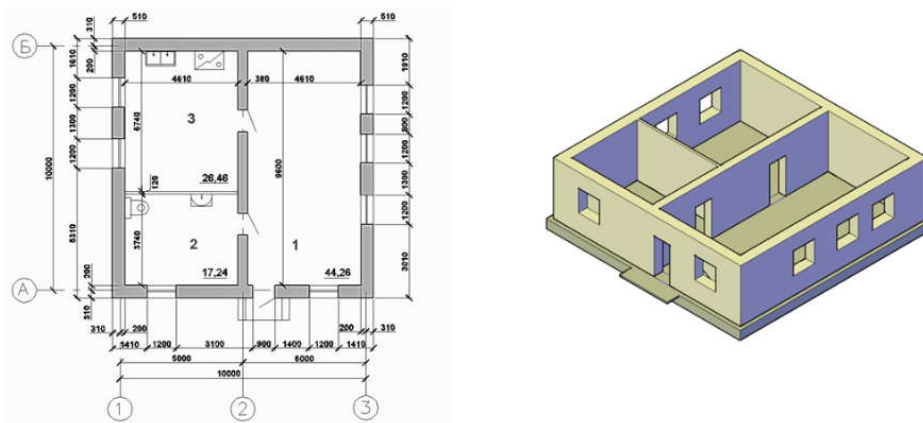
Рисунок 2 – Подготовка плана здания в графическом редакторе AutoCAD
