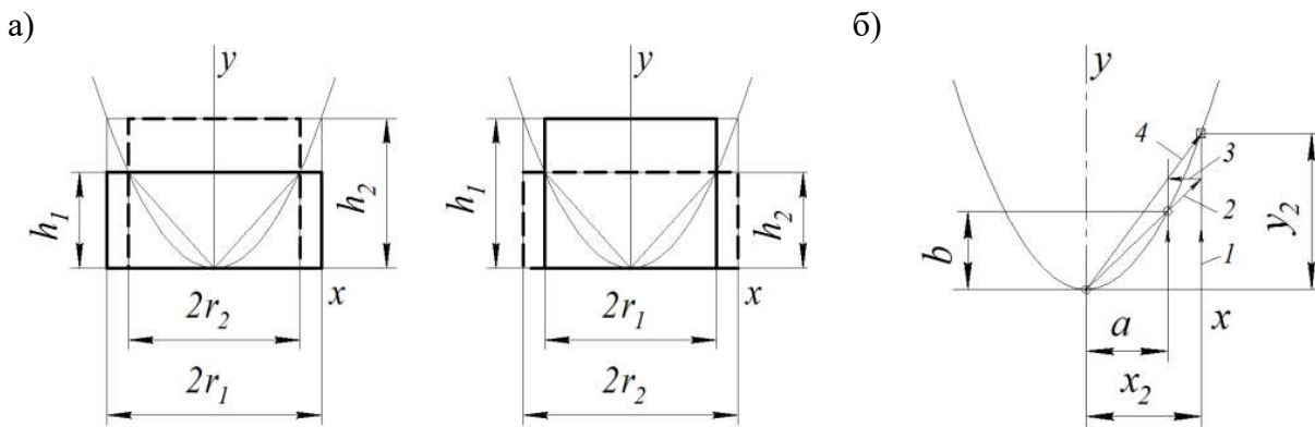
Рисунок 2 – Эквиобъемное преобразование цилиндра в цилиндр (а), построение точек параболы (б) – парабола показана для наглядности
