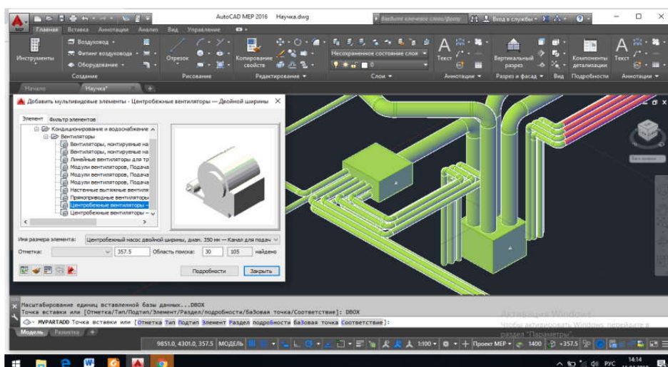
Рисунок 2 – Подсоединение оборудования
