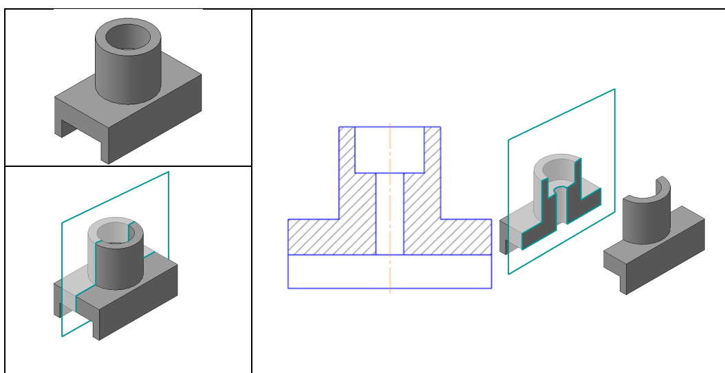
Рисунок 2 – Формирование понятия «разрез»
