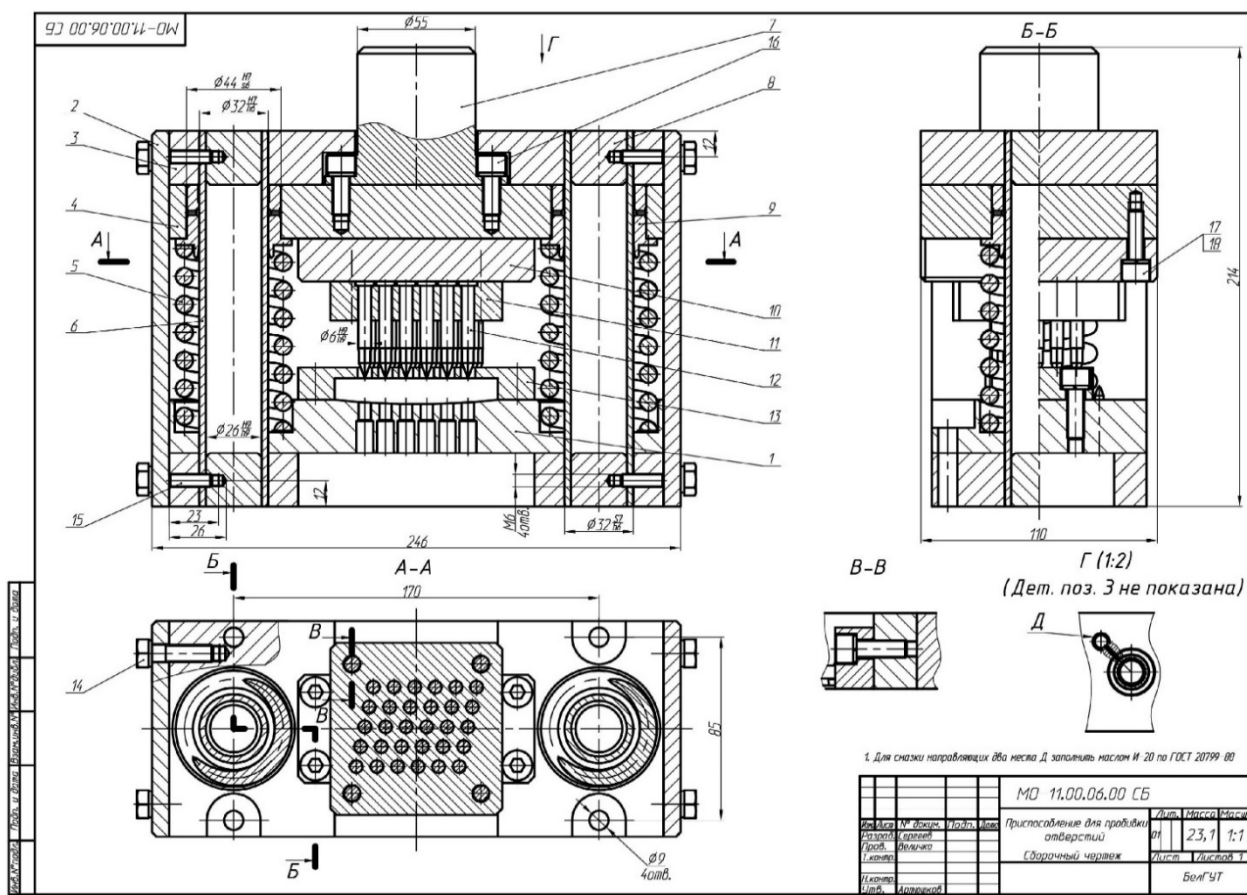
Рисунок 2 – Сборочный чертеж приспособления
