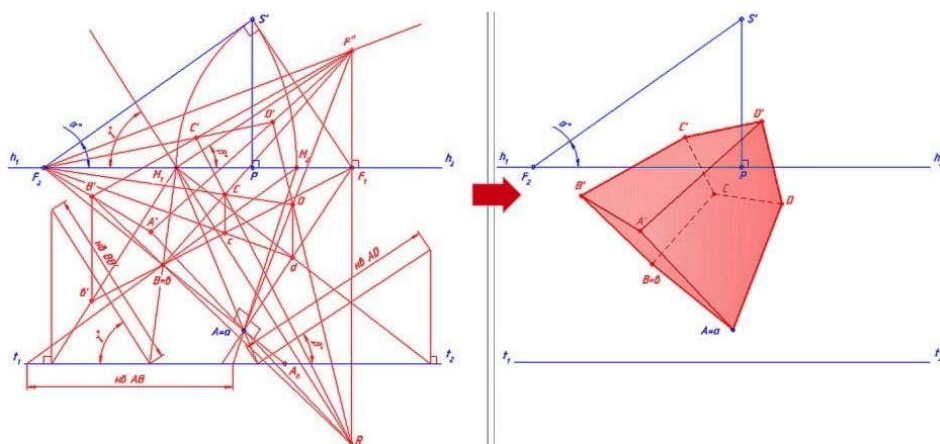
Рисунок 2 – Дополнительные слои для проверки задания: линии построения и результат построения
