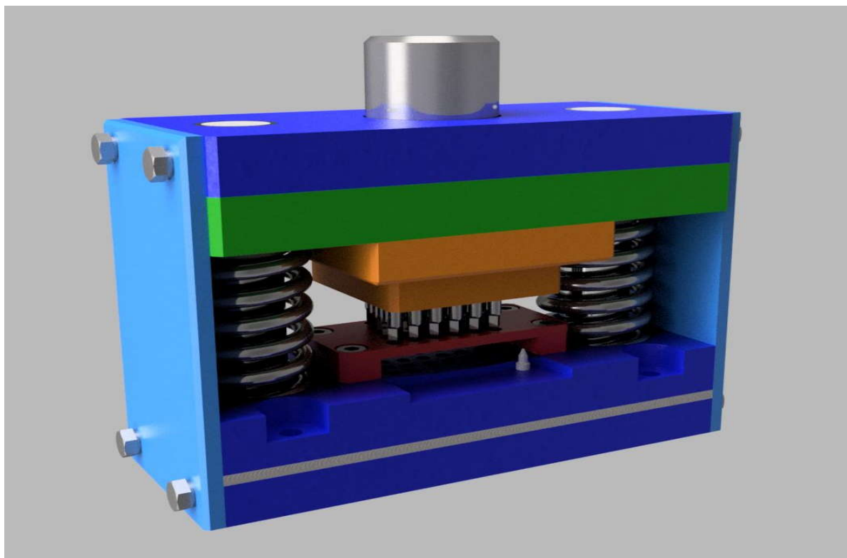
Рисунок 1 – Трехмерная модель приспособления
