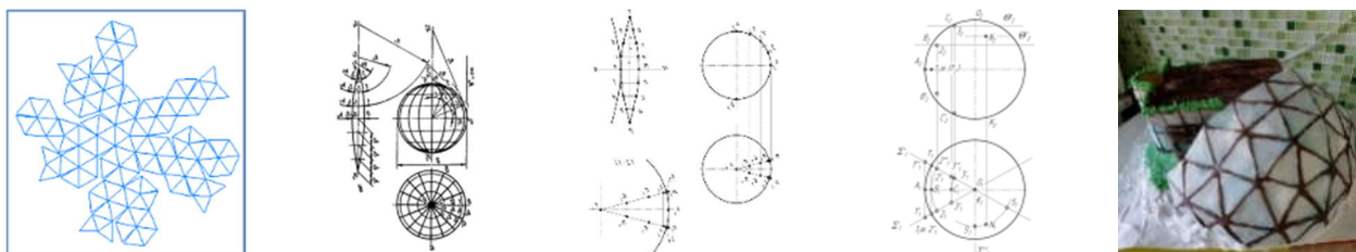
Рисунок 2 – Развертка сферы методом триангуляции, рассечением меридианными плоскостями, приближенная развертка, развертка полуцилиндра, макет купола
