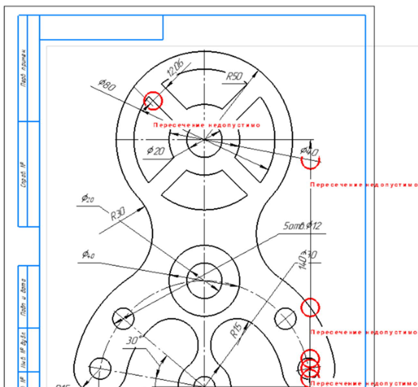
Рисунок 3 – Этап 3 – проверка тестового чертежа № 2 на правильность размещения размерных линий
