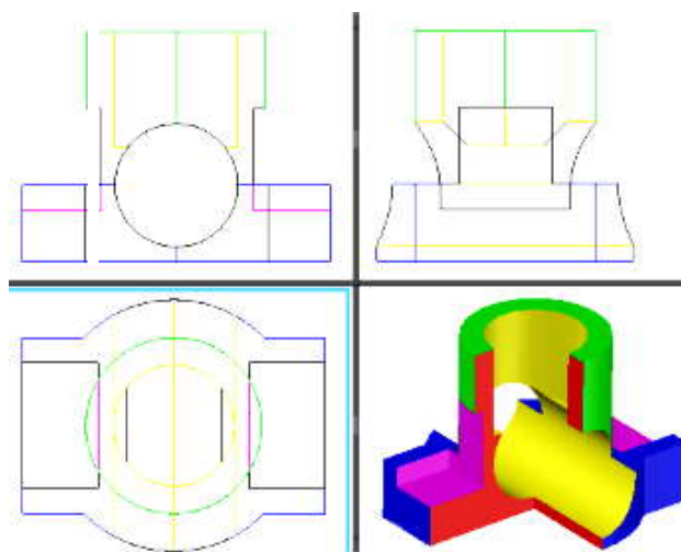
Рисунок 3 – Пример построения чертежа по модели
