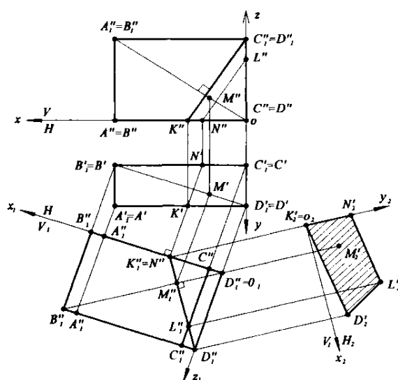
Рисунок 1 – Решение задачи на проекциях
